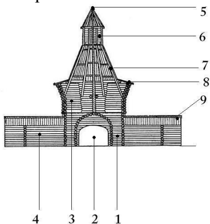
Рис. 6 Чертеж воротной башни Николо-Карельского монастыря XVII века: 1 – четверик; 2 – воротный проем; 3 – восьмерик; 4 – боковой придел; 5 – колпак; 6 – дозорная будка; 7 – шатер; 8 – полица; 9 – двухскатная кровля придела.
