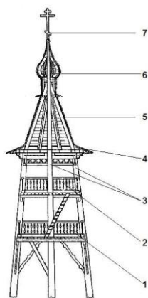
Рис. 9 Чертеж пятистолбчатой колокольни из с. Кижма XVIII века: 1- галерея; 2 звонница; 3 – несущие столбы; 4 – полица; 5 – шатер; 6- глава; 7 – крест.
