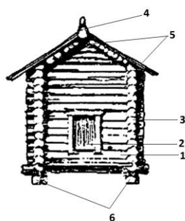
Рис. 8,11,12 Амбар, келья, четырехстенная избушка: 1- венец; 2 – дверной проем; 3 – соединение бревен в срубе с остатком; 4 – конек; 5 – кровля двухскатная; 6 – опоры
