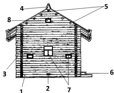
Рис.10 Чертеж дома четырехстенка: 1- окладник; 2 – отдушина; 3 – соединение бревен в срубе с остатком; 4 – конек; 5 – кровля двухскатная; 6 – крыльцо 7 – красное и волоковое окно 8 – самцовое окно
